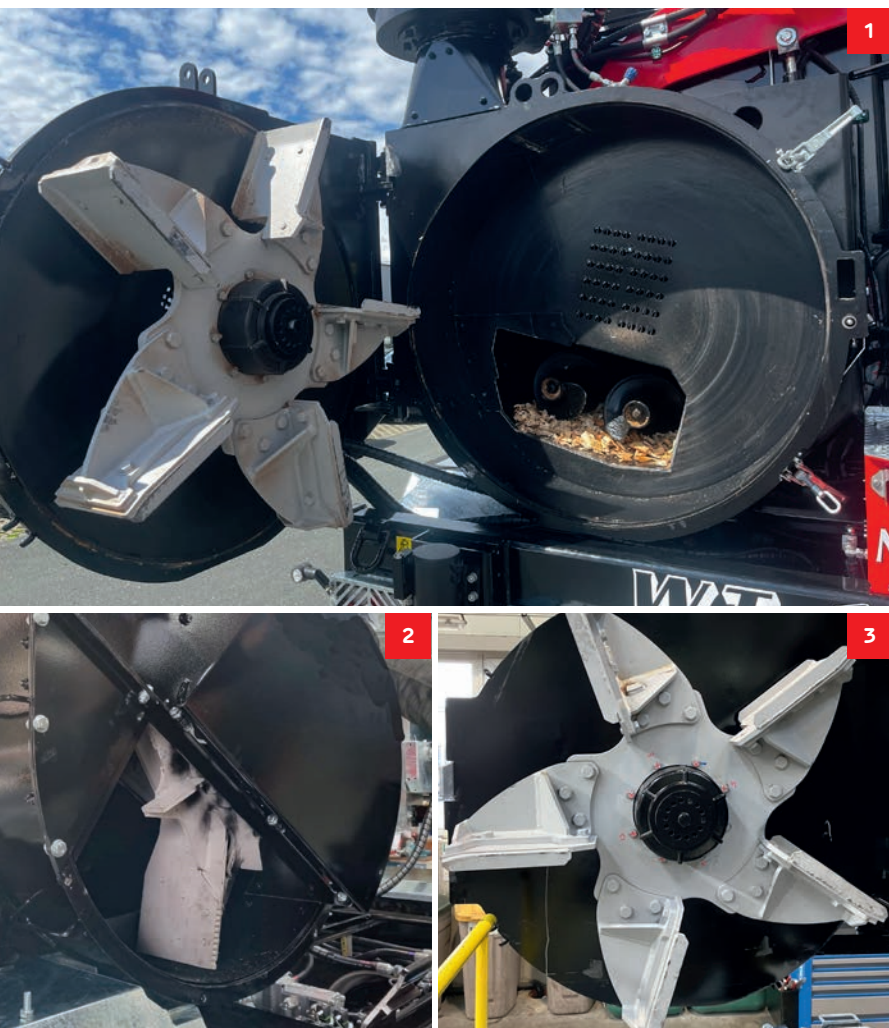
1. Hydraulisches Gebläse mit schwenkbarem Gebläsedeckel 2. Mechanisches Gebläse (Optional mit Industriefreilauf) 3. Neu entwickelter MUS-MAX Hochleistungs-Gebläseflügel
